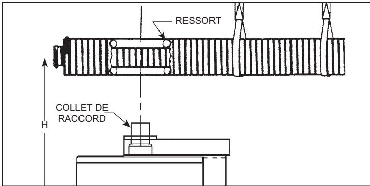
Figure 3E - Comment étirer le conduit de ventilation.
