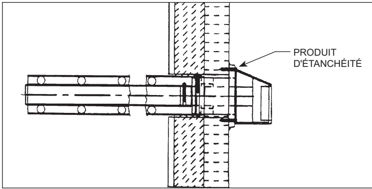
Figure 3D - Fixation de la terminaison au mur extérieur.
