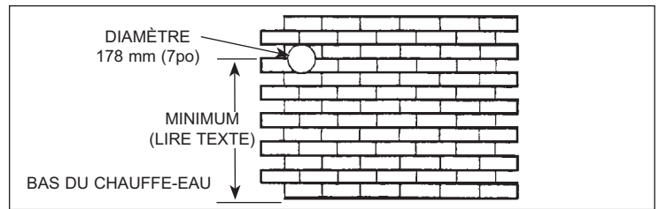
Figure 3A - Choix de l'emplacement de la terminaison.
