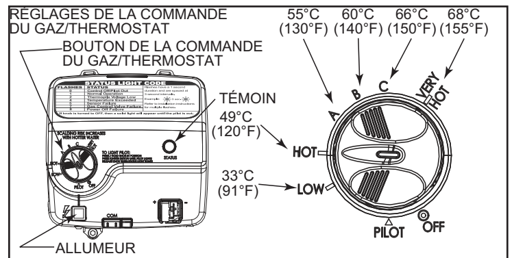
Figure 26 - Réglages de la commande du gaz/thermostat
