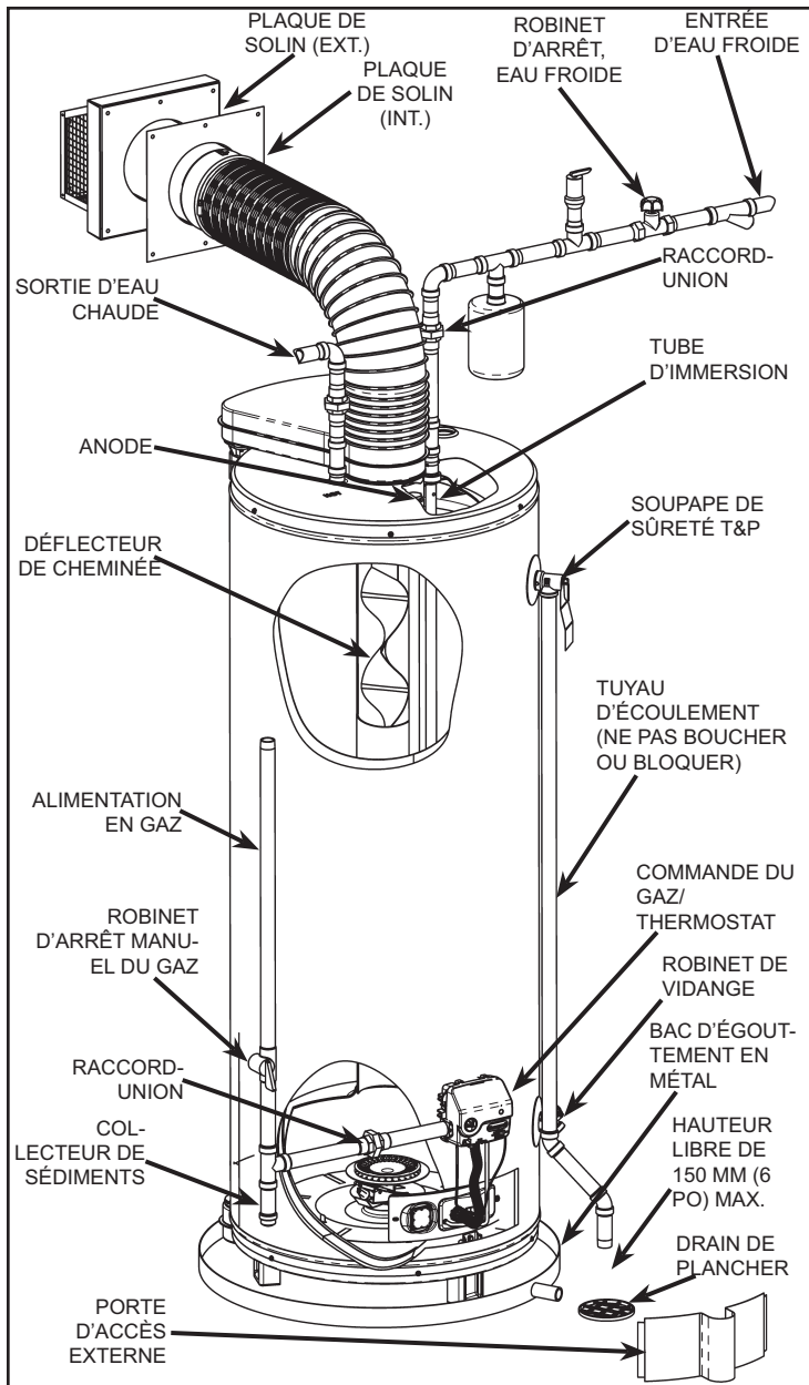
Figure 2A - Composantes d'installation.
