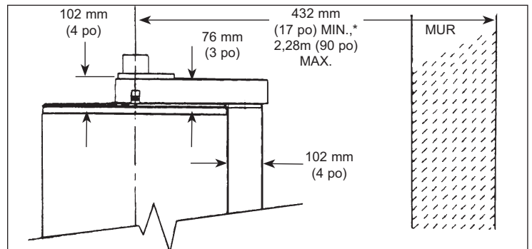
Figure 3B - Positionnement du chauffe-eau à son emplacement final.
