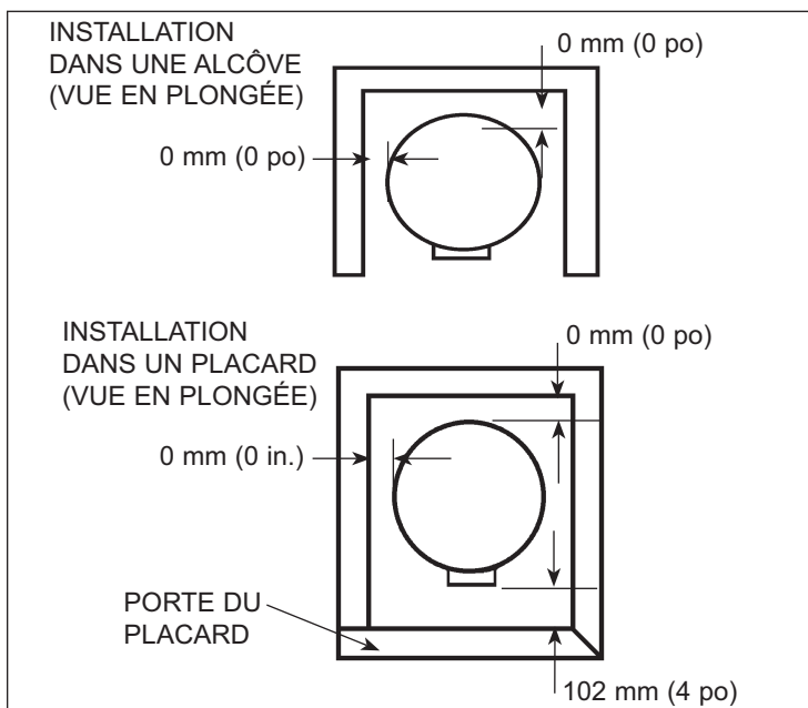
Figure 1 Distances de dégagement minimales
