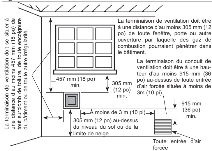
Figure 3 - Restrictions sur l'emplacement de la terminaison
