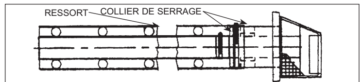
Figure 3C - Système d'évacuation spécial.
