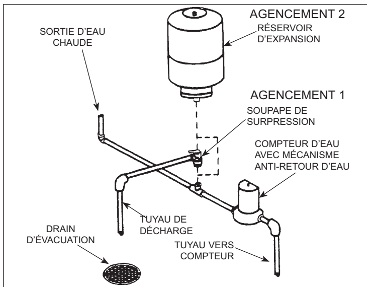
Figure 2B - Composantes optionnelles.
